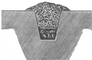
□ Рис. 5. Дренаж из мелкой гальки Дренажные трубы кладутся на дно узких канавок, вырытых узкими лопатами, и засыпаются обратно вынутой из канавок землей.
